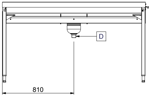
Zij aanzicht
